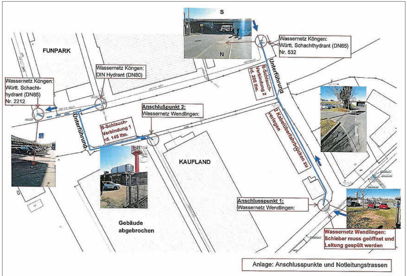
Lageplan Anschlusspunkte und Notleitungstrassen
